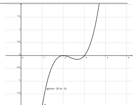
Figura 2: Gráfico da função g(x) = x^3 - 7x^2 + 16x - 12
