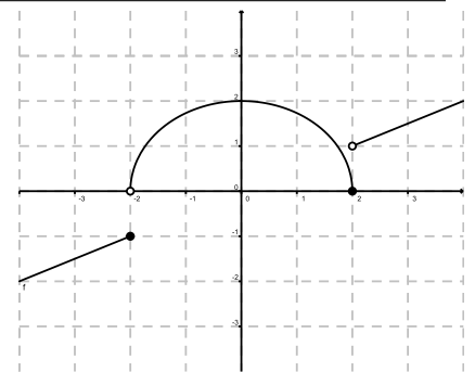
Figura 1: Gráfico de g(x)
