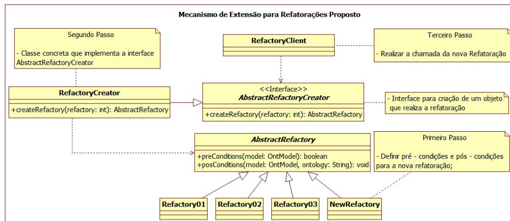
Figura 49: Mecanismo de extensão de refatorações
