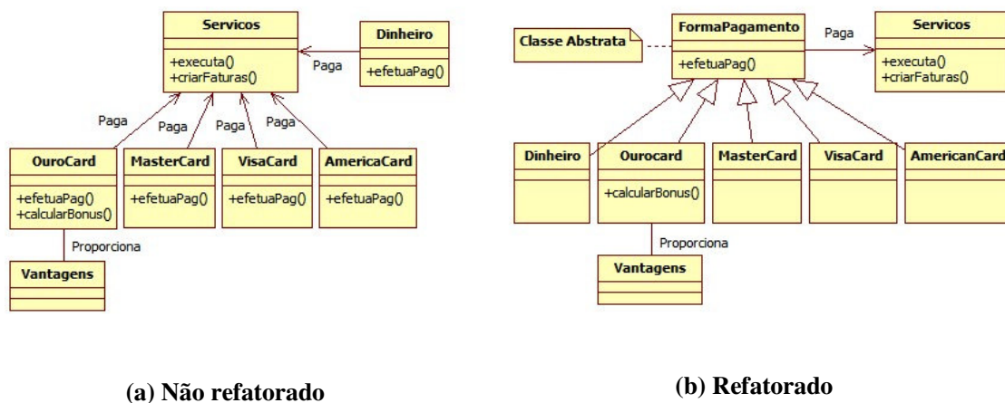
Figura 54: Primeiro caso do padrão criar classe abstrata
