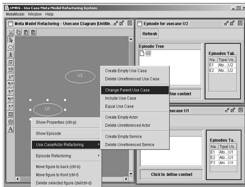
Figura 22: Aplicação de uma refatoração de caso de uso (XU, J., 2004)
