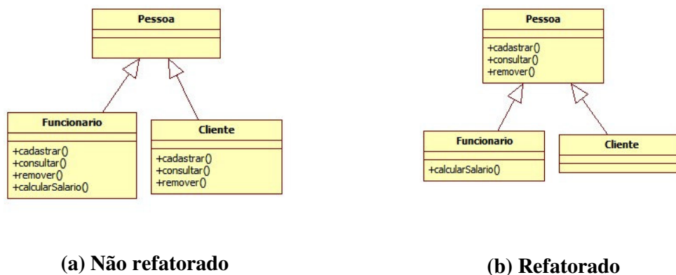
Figura 52: Subir método na hierarquia
