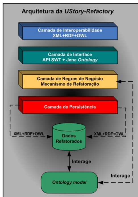
Figura 25: Arquitetura da UStory-Refractory
