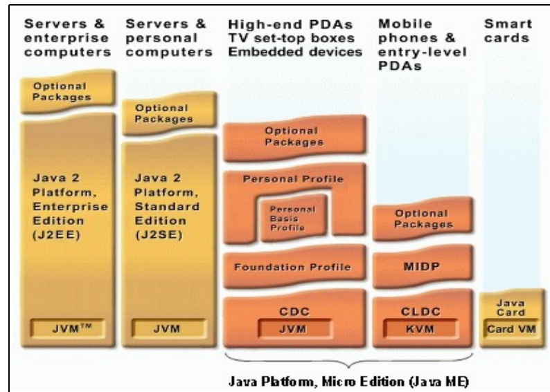
Figura 18: Plataforma Java [SUN 2008].
