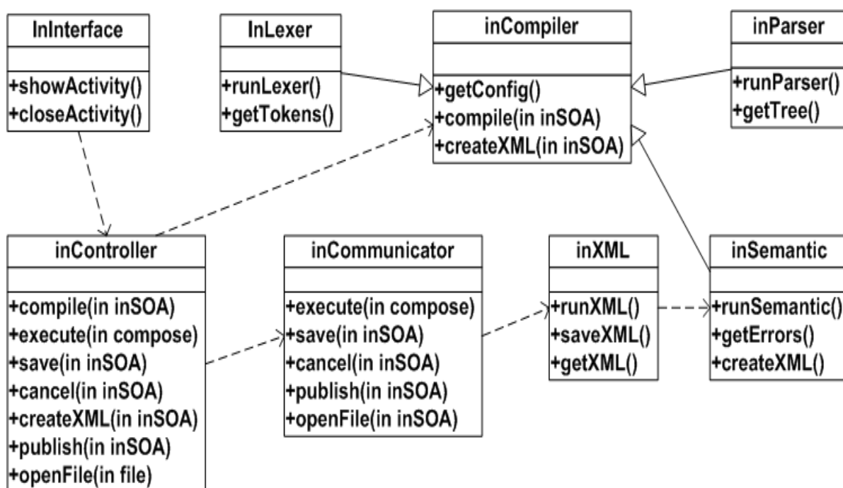
Figura 32: Diagrama de classes das principais classes.
