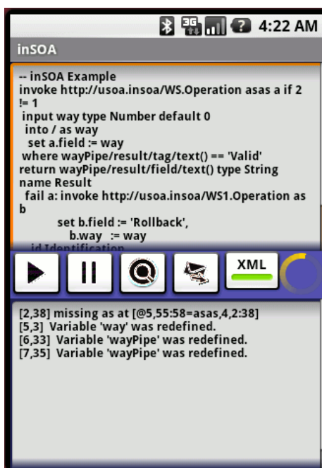
Figura 37: Tela com os erros de compilação do inSOA.
