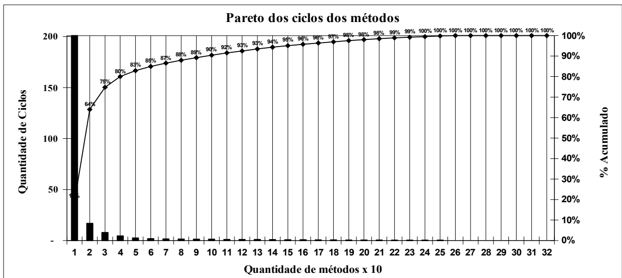
Figura 44: Pareto dos ciclos dos métodos do compilador inSOA .
