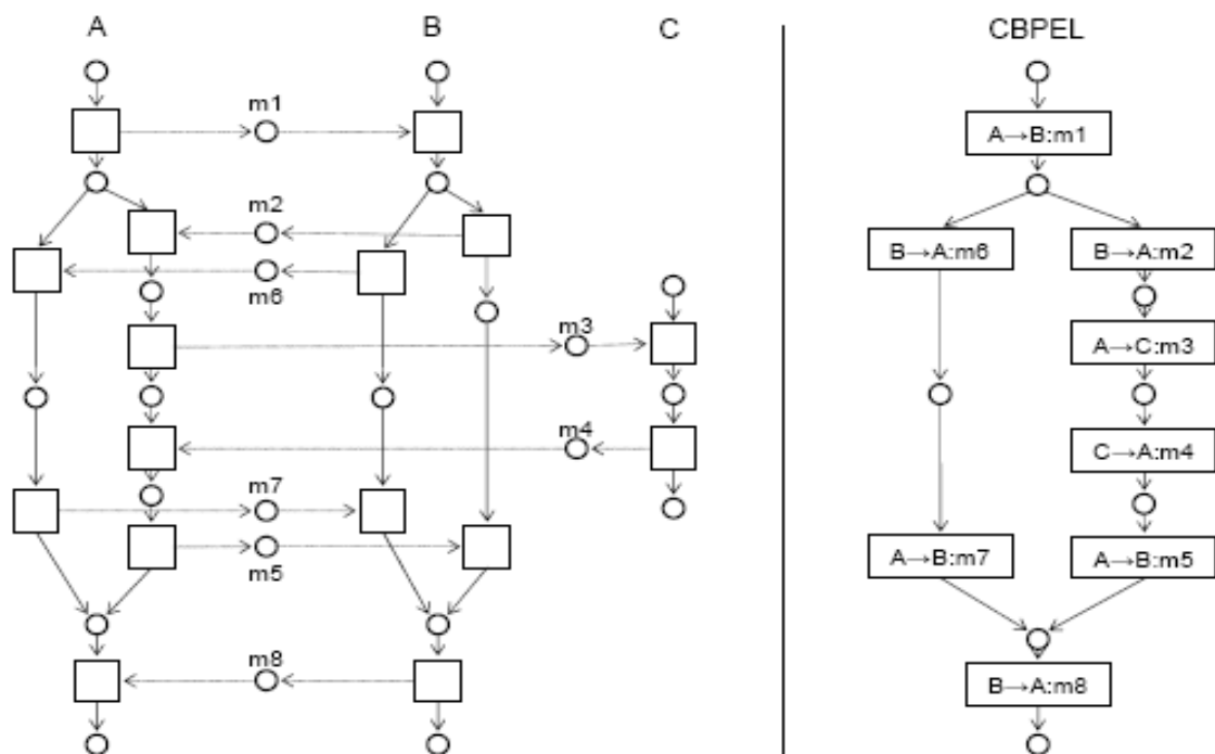
Figura 20: Exemplo de forma global unificada utilizando uma decisão ( switch ) [Teófilo 2005].
