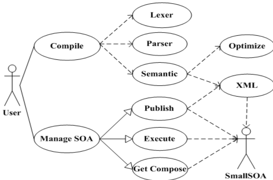
Figura 29: Diagrama de caso de uso da inSOA .
