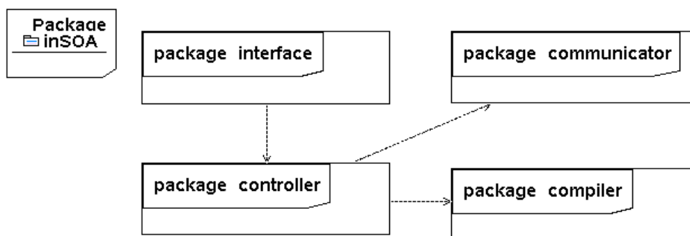
Figura 31: Diagrama de Pacotes.
