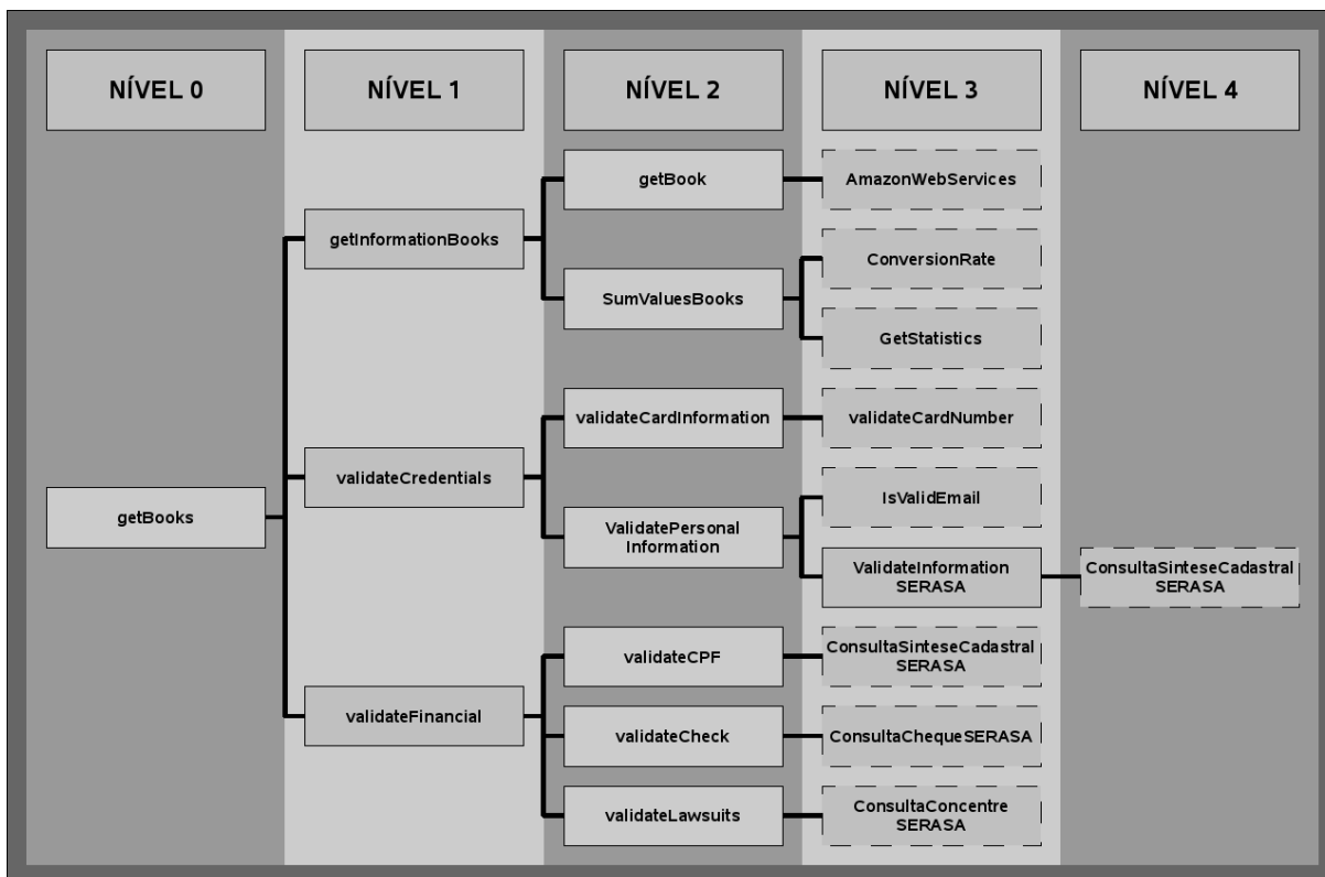
Figura 42: Cenário I - Consulta de Livros.
