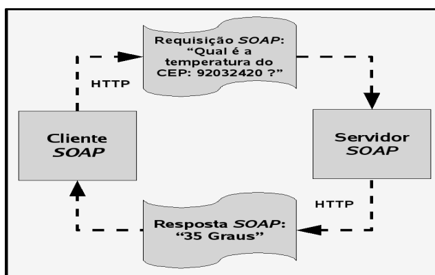
Figura 6: Funcionamento do serviço SOAP de temperatura por CEP do XMethods.net.
