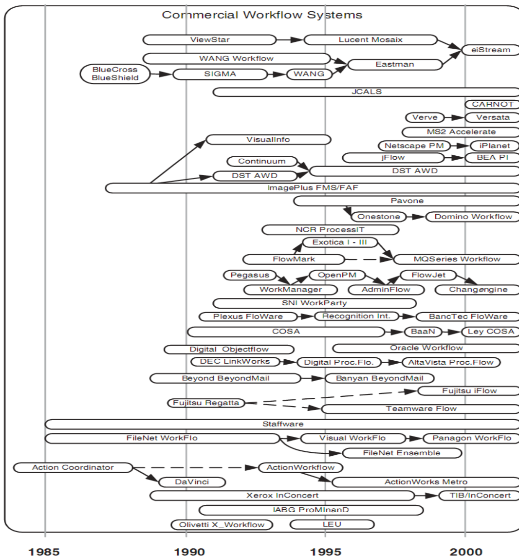
Figura 11: Automação de processos e sistemas de workflow [Mühlen 2002].
