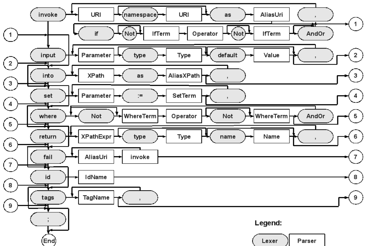
Figura 28: Diagrama da sintaxe da linguagem inSOA .
