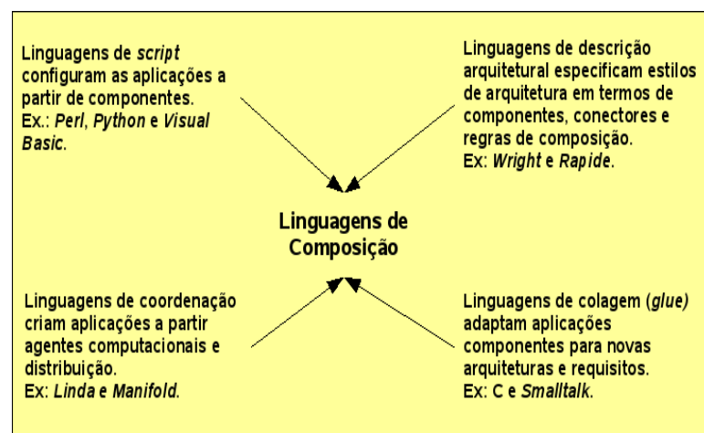
Figura 21: Conceitos chaves das linguagens de composição de componentes. Adaptado de [Archemann 2001].
