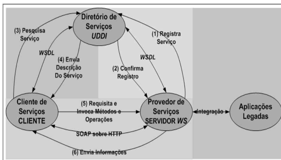
Figura 4: Modelo de referência WS. Adaptado de [W3C 2004].
