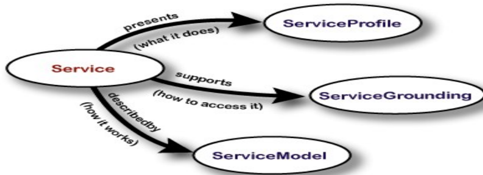
Figura 13: Serviços de ontologia da OWL-S [Martin 2004].
