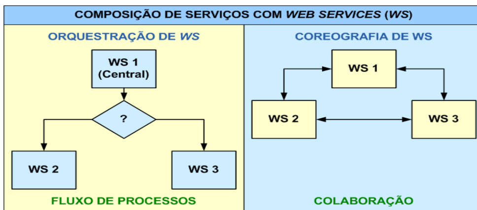
Figura 10: Composição de serviços WS por orquestração e coreografia.
