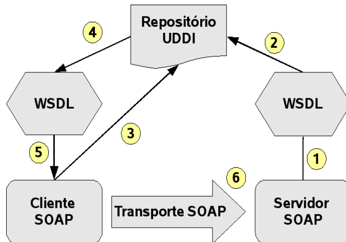
Figura 8: Uso do UDDI para descobrir um WS [Newcomer 2002].
