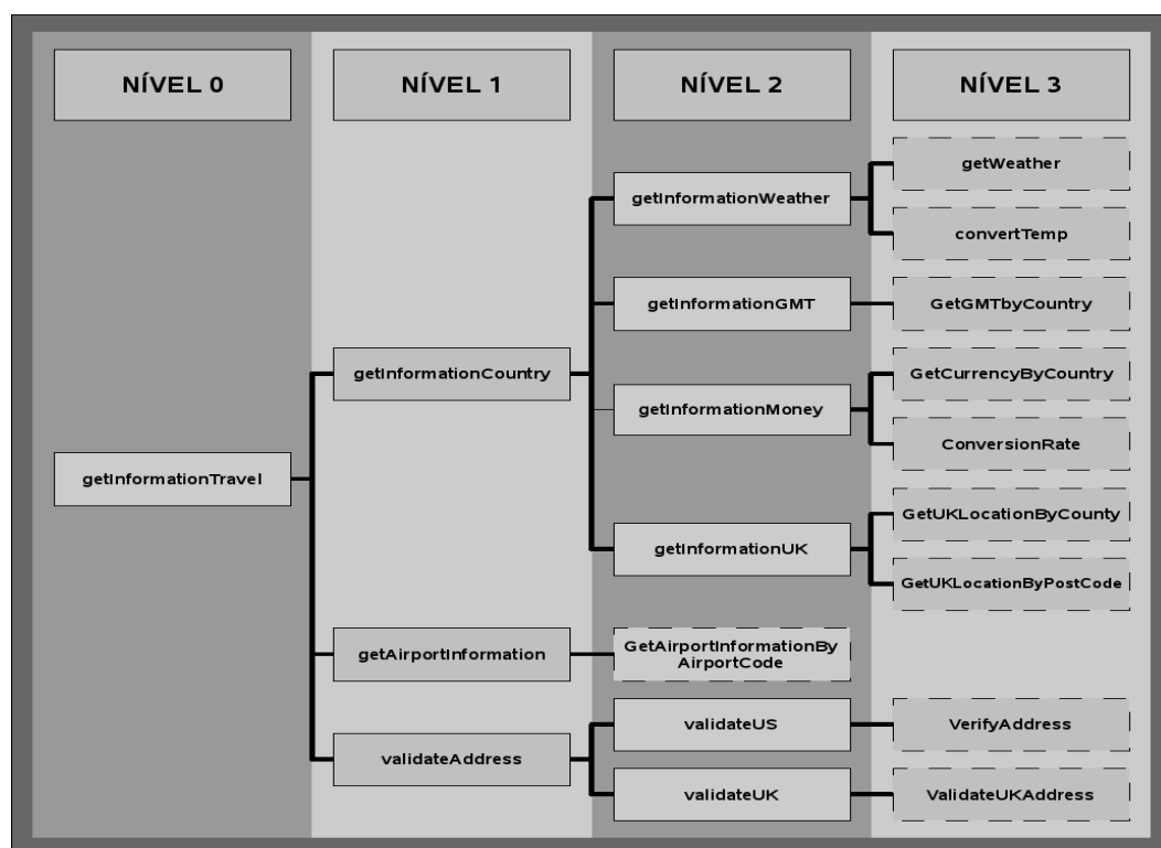
Figura 39: Consulta de Viagem.
