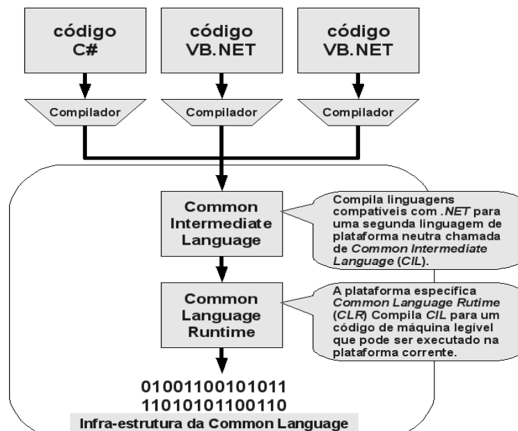
Figura 17: Infra-estrutura da CLR [MSDN 2008].
