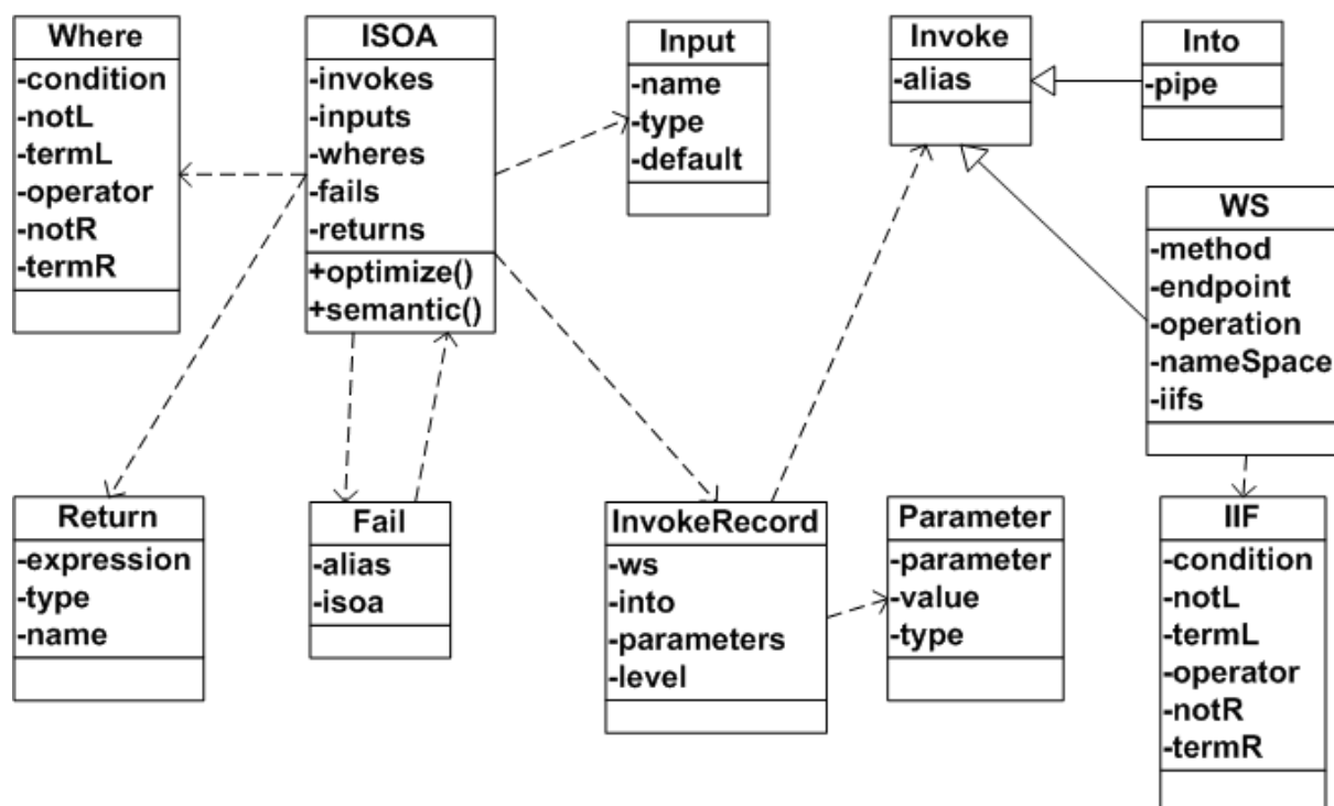
Figura 36: Diagrama de classes do objeto iSOA .
