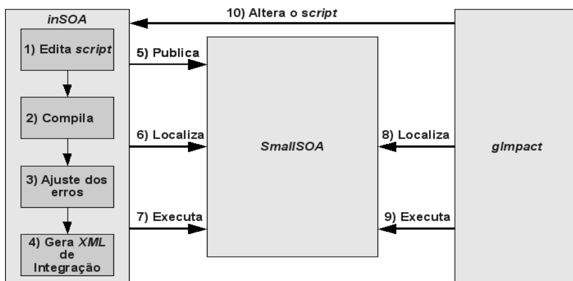
Figura 38: Processo do Estudo de Caso.
