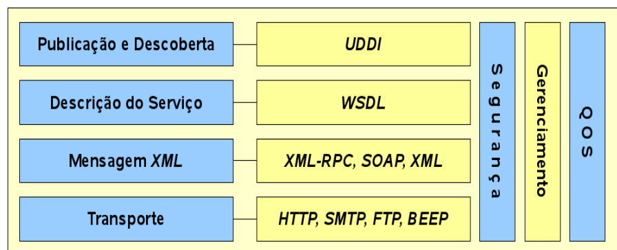
Figura 5: Modelo WS em camadas. Adaptado de [Cerani 2002].
