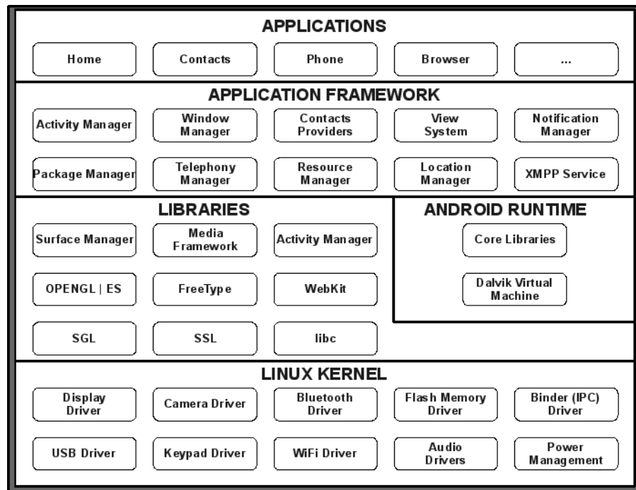
Figura 19: Arquitetura Android [Android 2008].
