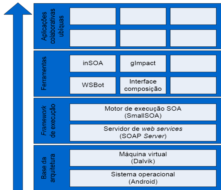
Figura 22: Arquitetura U-SOA.
