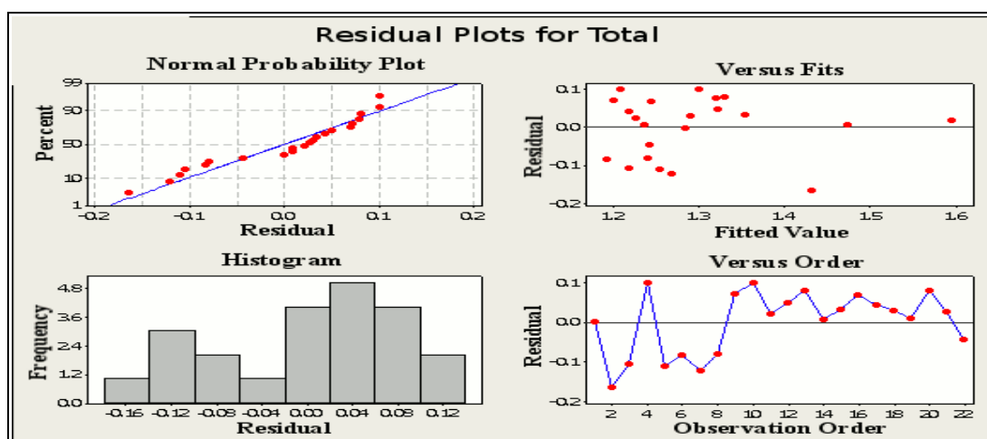
Figura 46: Gráfico de probabilidade normal.
