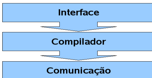
Figura 30: Camadas inSOA .
