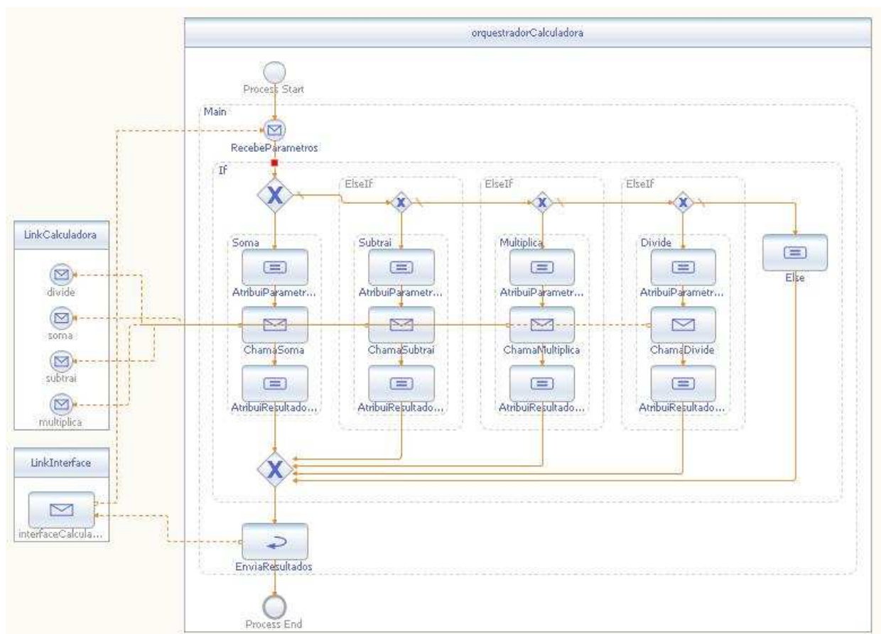
Figura 2.14 – Orquestração BPEL
