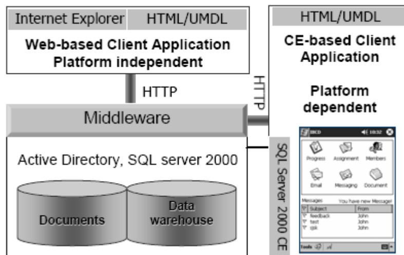
Figura 3.6 - Arquitetura de um Sistema Colaborativo Móvel
