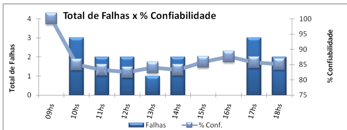
Figura 5.5 – Gráfico Total de Falhas x % Confiabilidade
