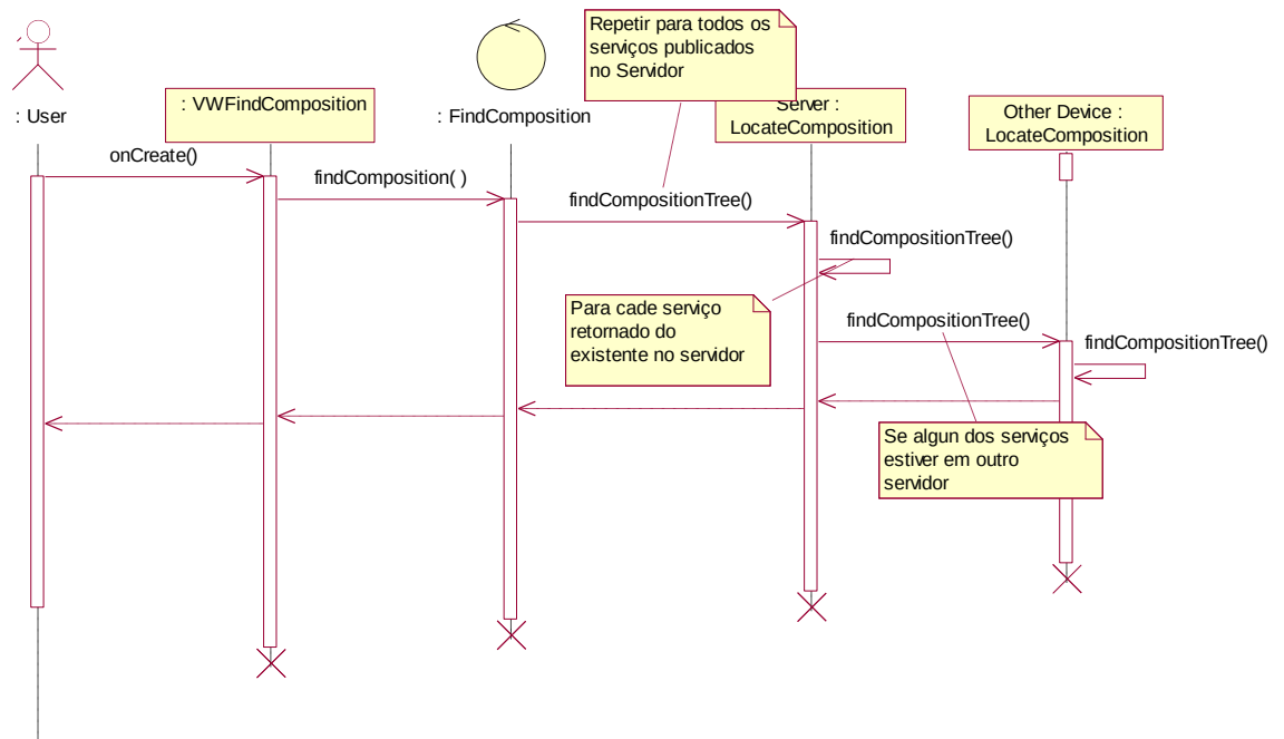
Figura 4.15 – Diagrama de Seqüência de Busca da Composição
