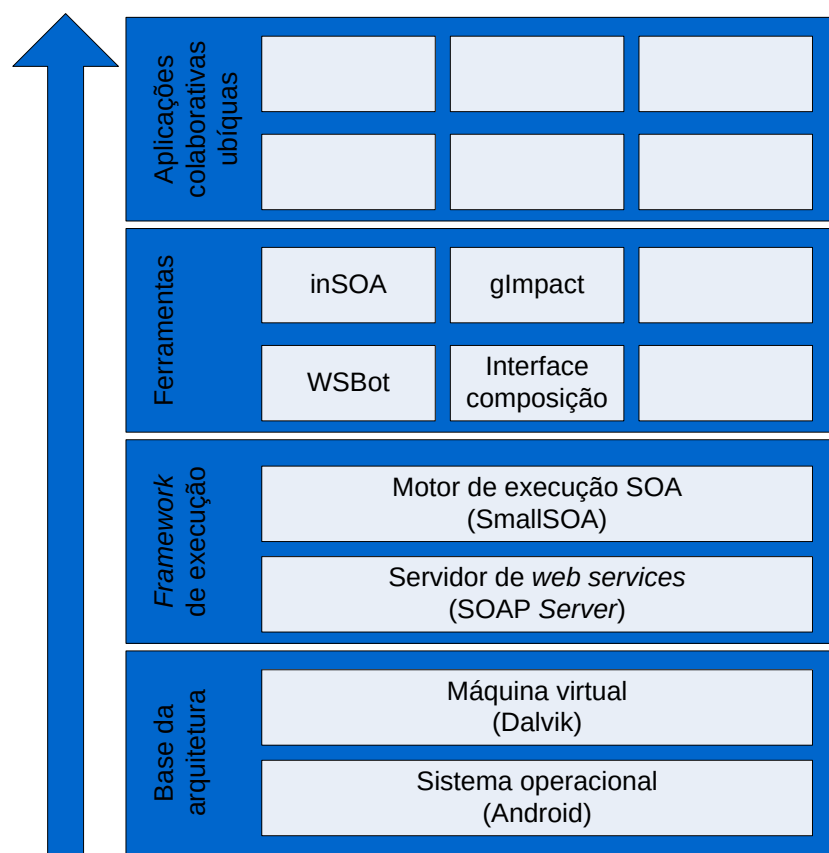
Figura 4.1 – Arquitetura U-SOA
