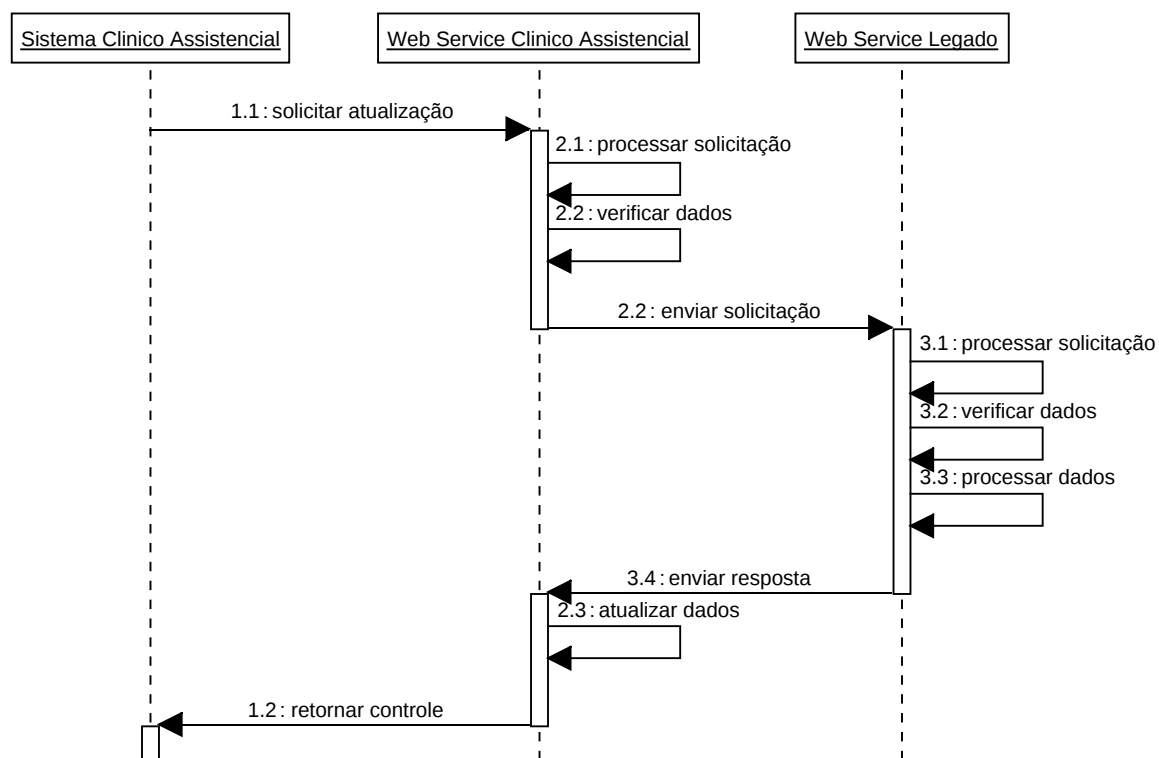
FIGURA 4.4 – Modelo de interações: diagrama de sequência.
