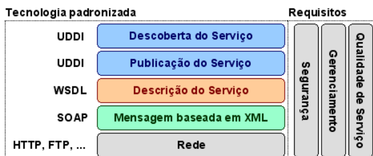
FIGURA 2.14 – Camadas conceituais de Web Services , adaptado de Hansen (2002, p. 3).
