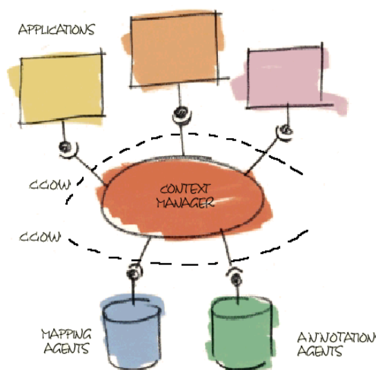
FIGURA 3.5 – Arquitetura CCOW (SELIGER, 2001).
