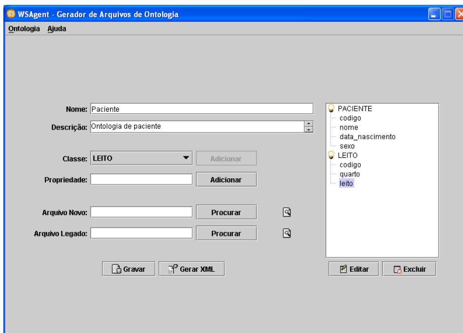
FIGURA 4.10 – Gerador de arquivos de Ontologia (modo de criação/edição).
