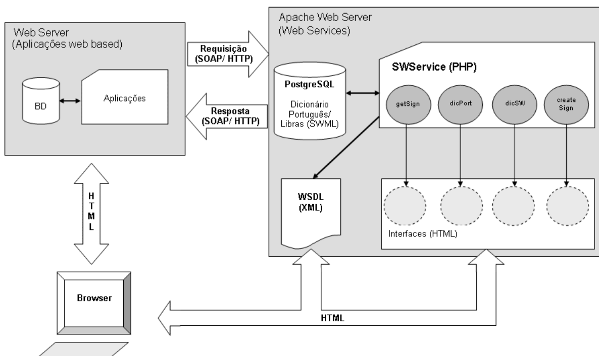
Figura 6.1 - Arquitetura de uso da biblioteca de serviços SWService
