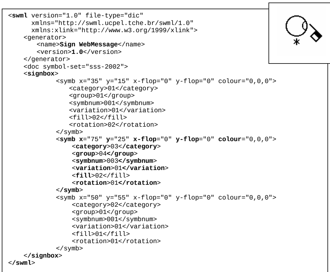
Figura 2.15 - Código SWML que descreve o sinal referente à palavra Surdo .
