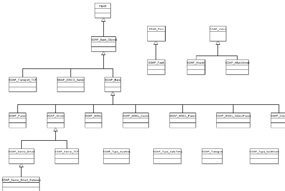
Figura 3.11 – Classes da PEAR SOAP
