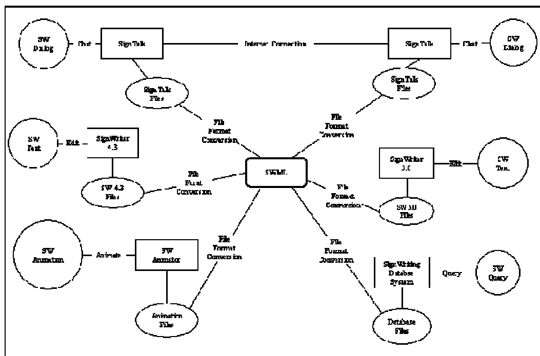
Figura 2.14 - Interoperabilidade através da SWML [COS 03]
