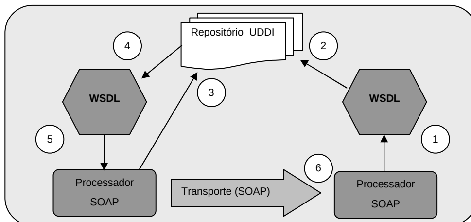
Figura 3.6 - UDDI utilizado para descobrir um Web Service [NEW 02]
