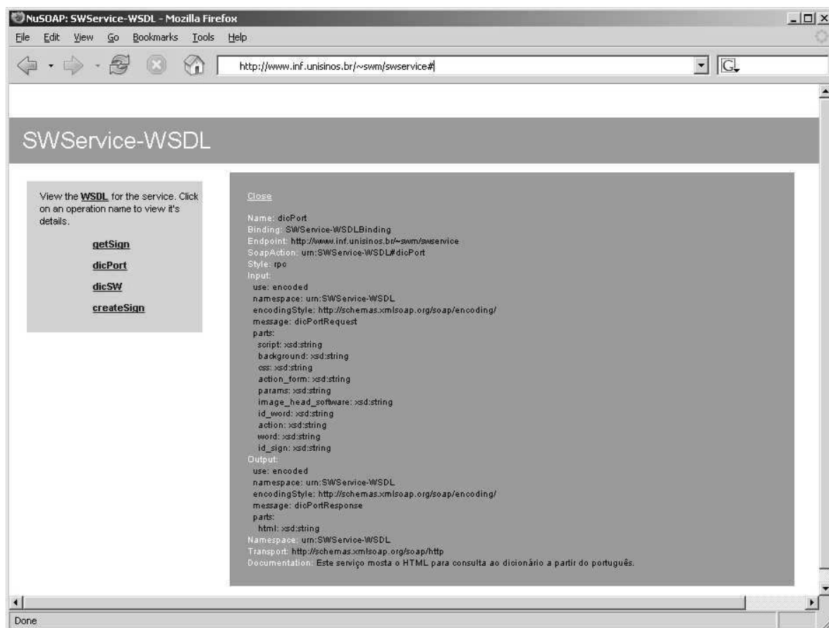
Figura 6.9 - Interface do serviço dicPort
