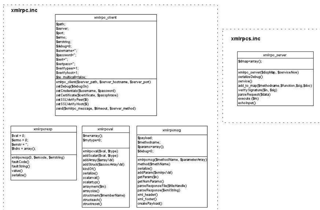
Figura 3.8 – Classes, atributos e métodos do XML-RPC tollkit
