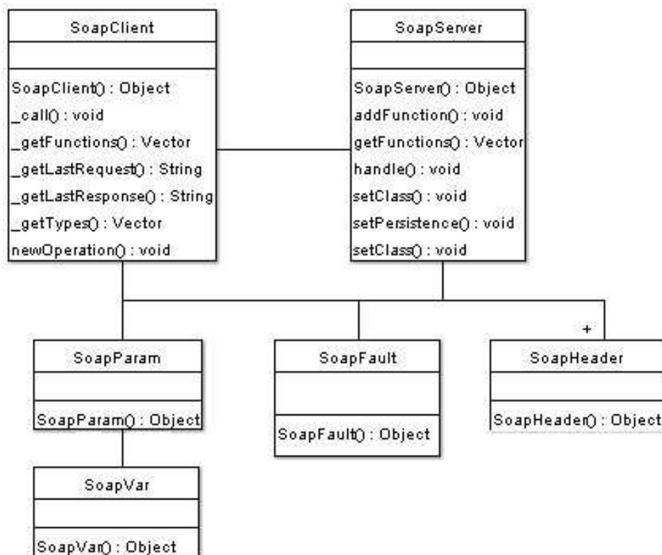
Figura 3.12 – Classes e métodos da SOAP Extension
