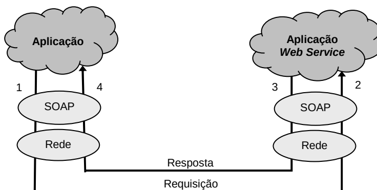
Figura 3.5 - Invocação do serviço utilizando SOAP [HAN 03a]
