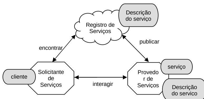
Figura 3.1 - Arquitetura dos Web Services [FER 03a]
