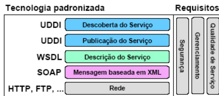
Figura 4.2: Camadas conceituais de Web Services (Rheinheimer, 2004).
