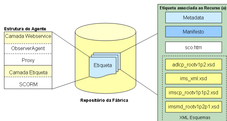
Figura 7.20: Estrutura da etiqueta da Fábrica de Adequação.
