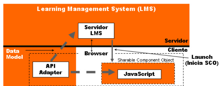
Figura 5.8: Run-Time Environment de uma plataforma de e-learning , adaptado de (SCORM, 2005).
