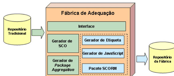
Figura 7.4: Serviços da Fábrica de Adequação.
