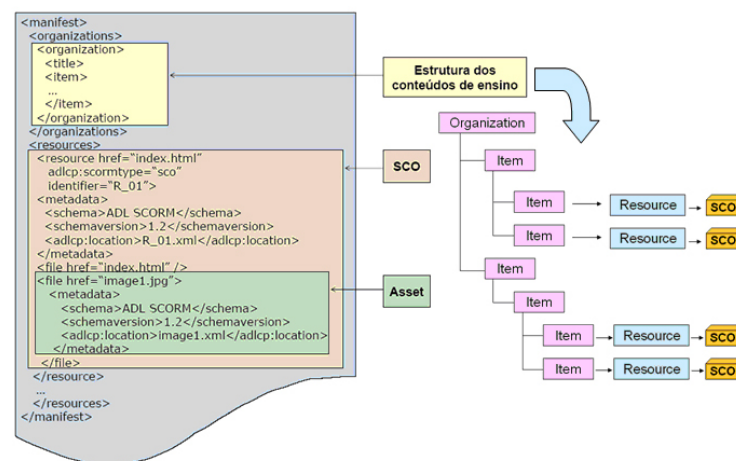
Figura 7.16: Manifesto de um Content Aggregation .
