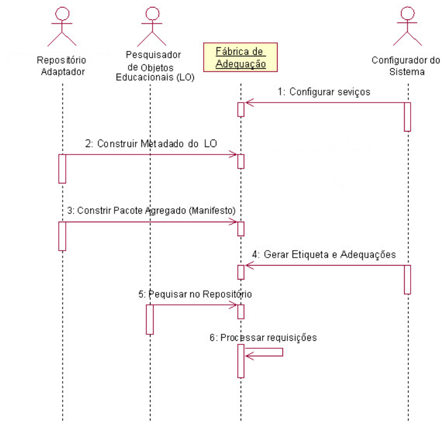
Figura 7.7: Diagrama de Sequência Geral da Fábrica.
