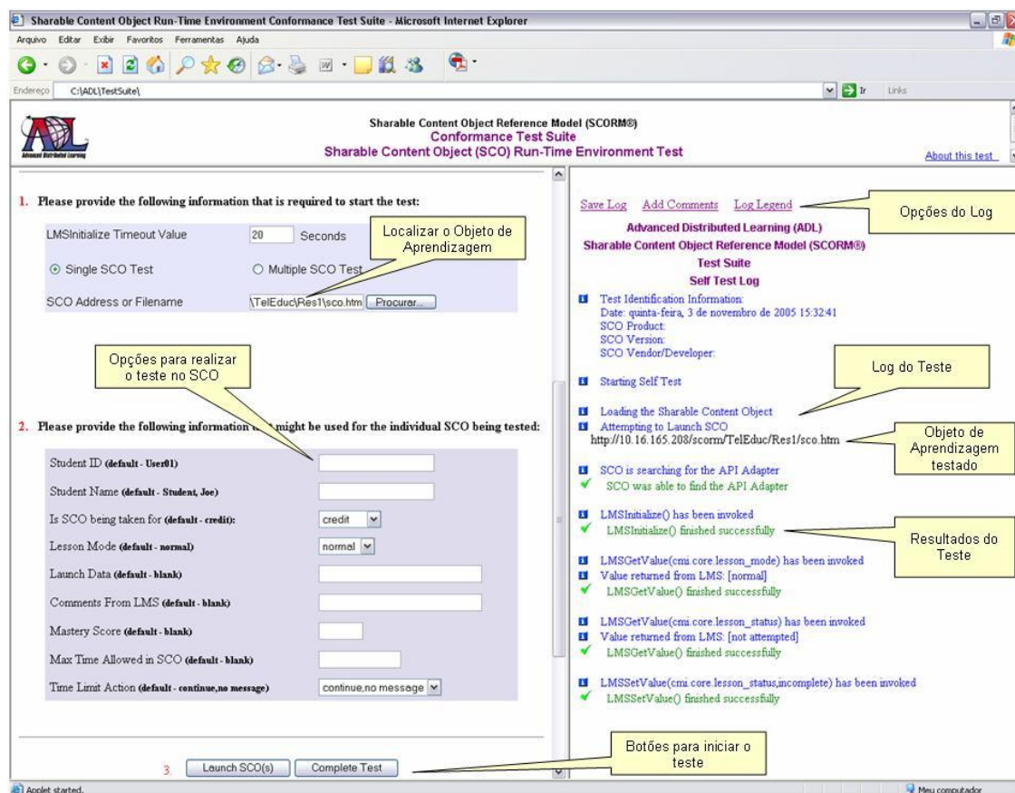
Figura 8.7: Exemplo de teste do Conformance Test Suite em um Objeto de Aprendizagem.
