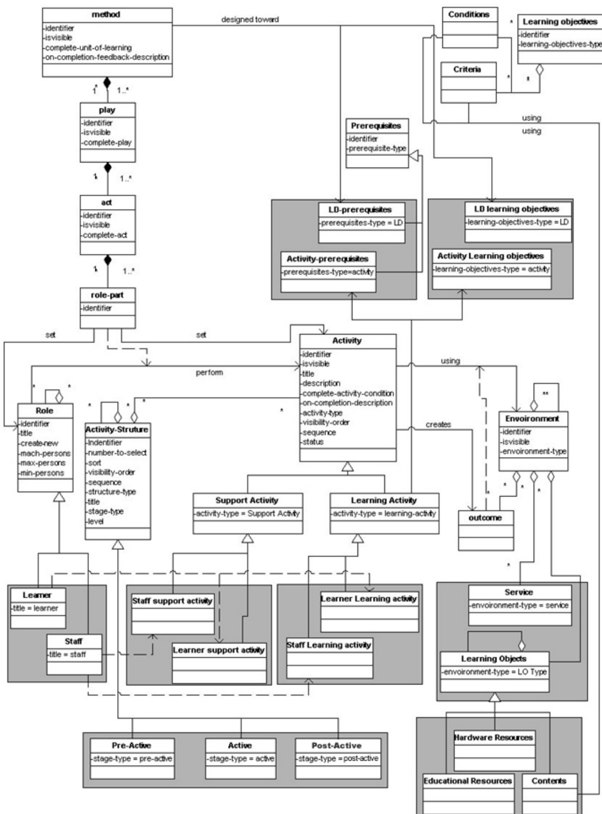
Figura 4.3: Ontologia de Design de Aprendizagem
