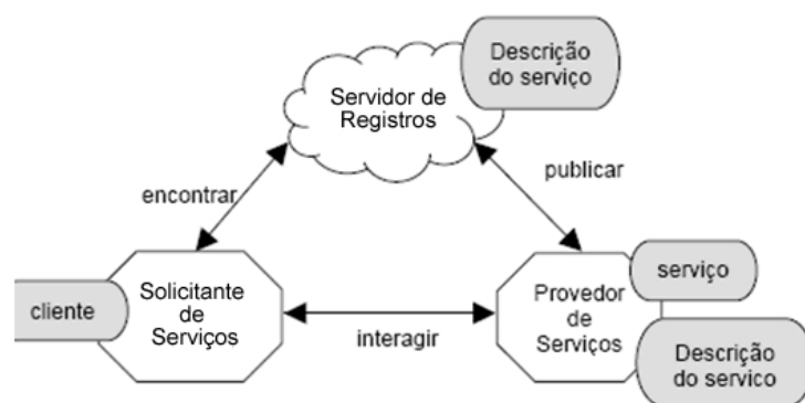
Figura 3.2: Arquitetura de Web services . (Ferris, 2003)
