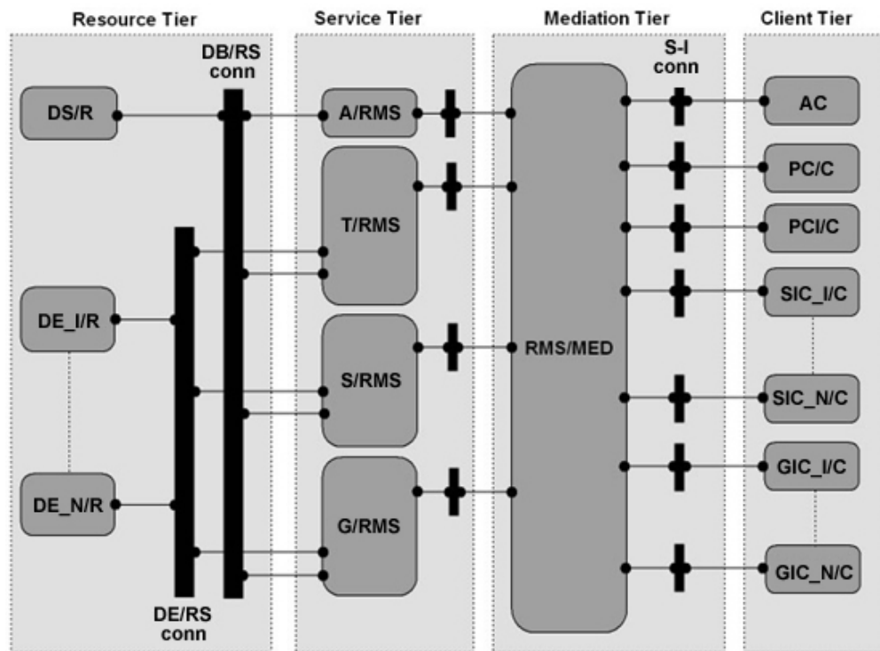
Figura 4.2: Arquitetura do Projeto EUME
