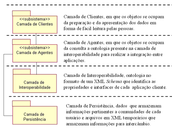
Figura 5.3: Funcionalidades resumidas das camadas WSMEL
