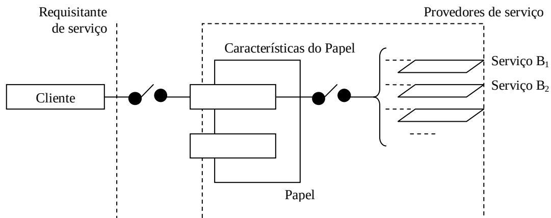
Figura 4.1 – Modelo do conector de serviço baseado em papel.
