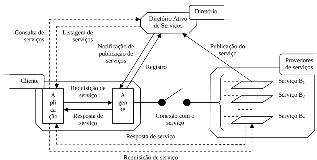
Figura 5.4 – Arquitetura de web services com suporte a composição dinâmica.
