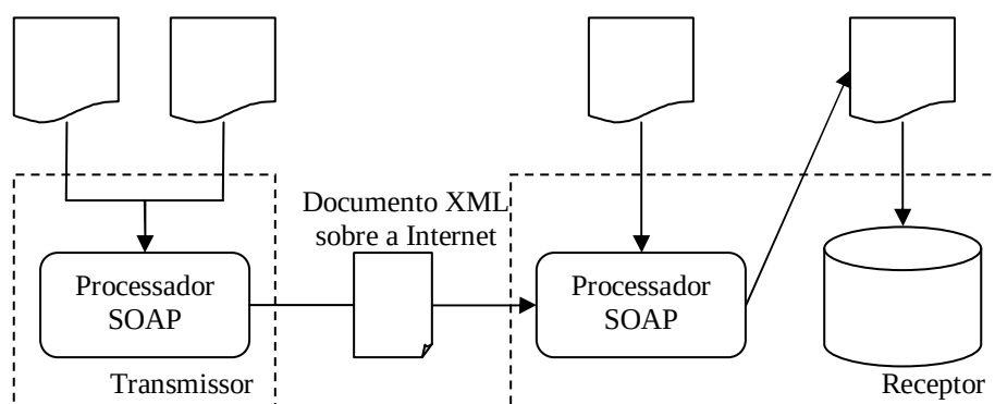
Figura 2.3 – Invocação de um web service . Adaptada de [Newcomer 02].
