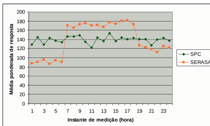
Gráfico 6.2 – Média ponderada de resposta do SPC e SERASA.
