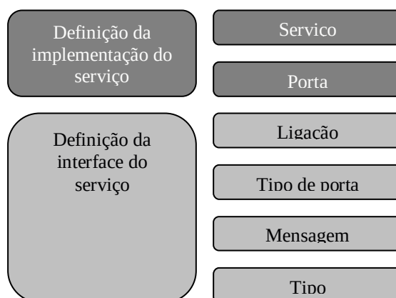
Figura 2.6 – Camada de descrição de serviços. Adaptada de [Souza 03].
