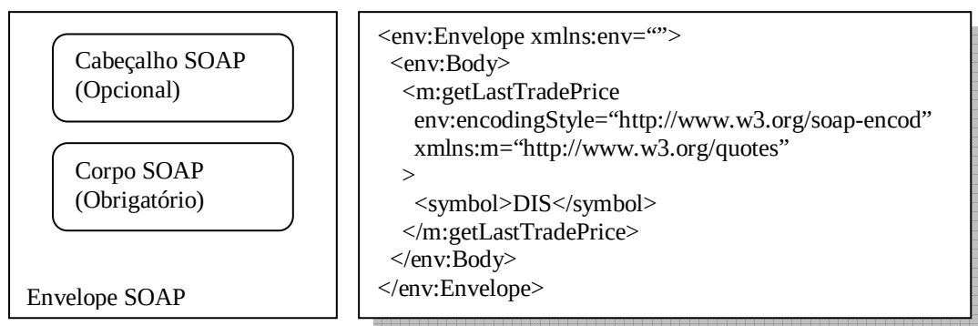
Figura 2.8 – Partes de uma mensagem SOAP [Scopel 05].
