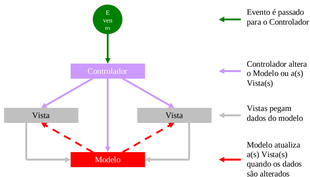
Figura 3.1 – Fluxo de controle do MVC.
