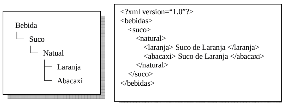
Figura 2.4 – Exemplo de uma hierarquia em XML.
