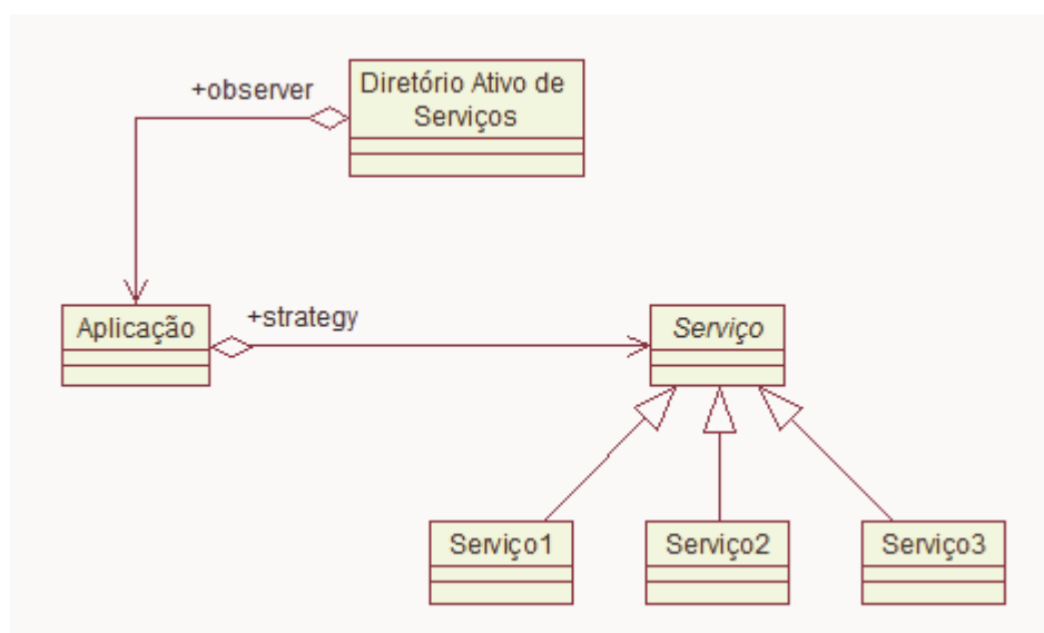
Figura 5.3 – Pseudo-arquitetura de web services com suporte a composição dinâmica baseada em padrões de projetos.
