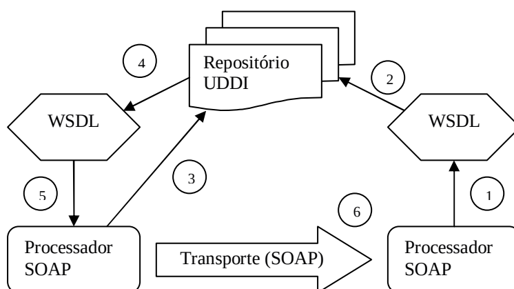
Figura 2.10 – UDDI utilizado para descobrir um web service [Newcomer 02].
