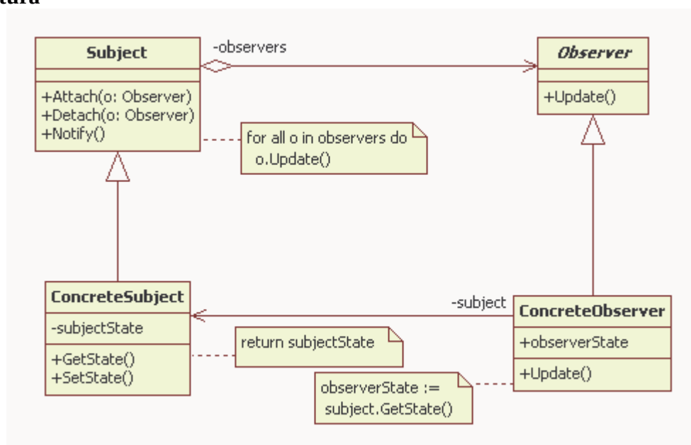
Figura 3.3 – Diagrama de classe UML do padrão observer [Shalloway 00].
