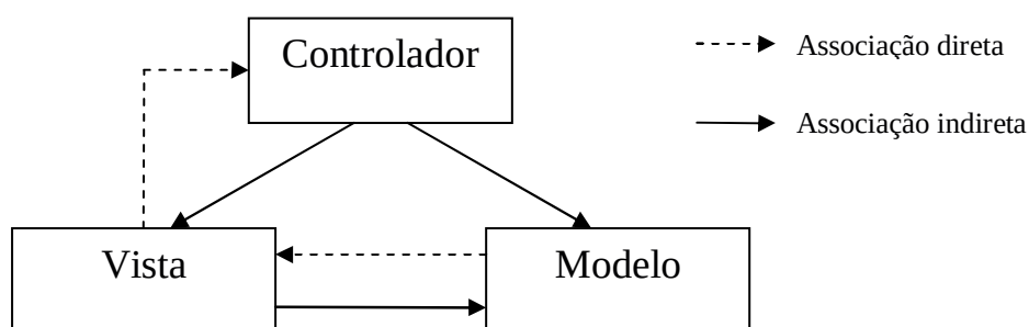
Figura 3.2 – Estrutura de relação entre os componentes do MVC.
