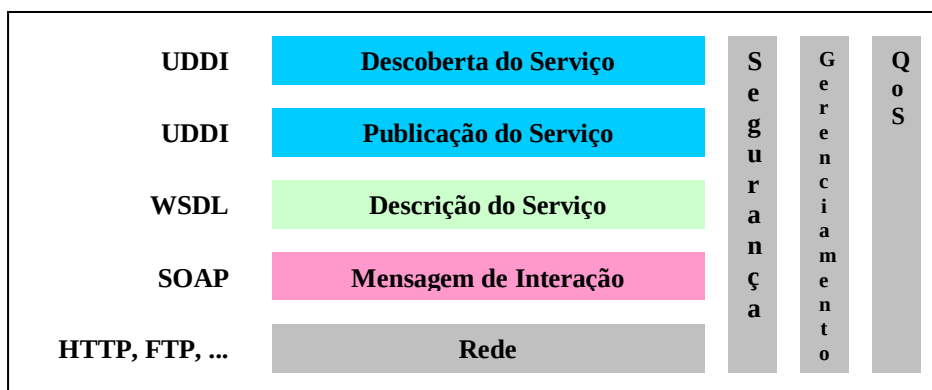
Figura 2.2 – Camadas conceituais de web services . Adaptada de [Rheinheimer 03].
