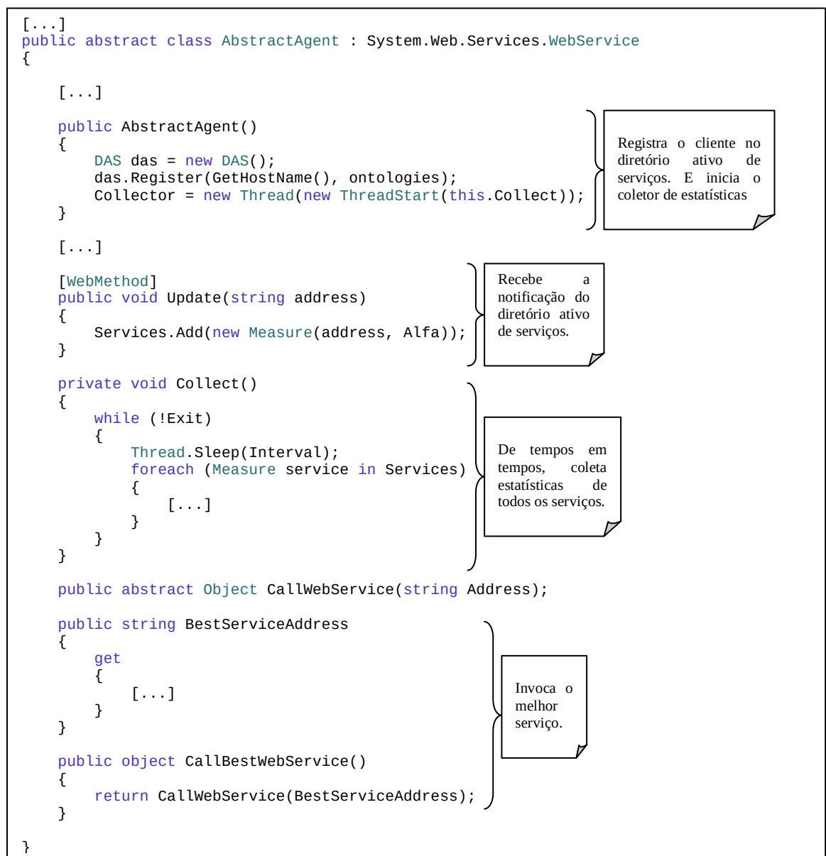
Figura 5.6 – Esqueleto de código do Framework do Agente.
