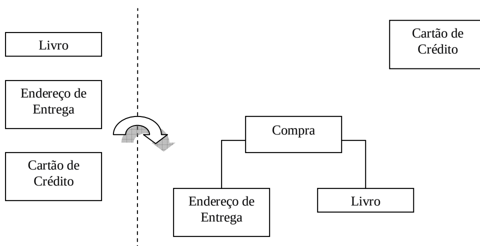
Figura 4.4 – Regra descrevendo a exigência mínima de um serviço requerido pelo cliente. Adaptada de [Hausmann 03].
