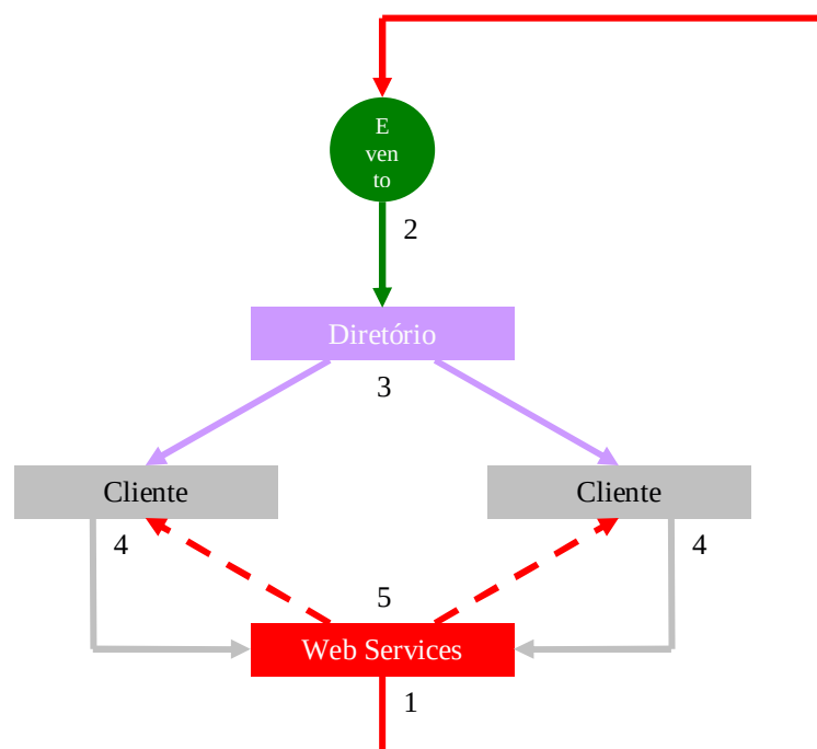
Figura 5.2 – Fluxo de controle de composição baseado no modelo MVC
