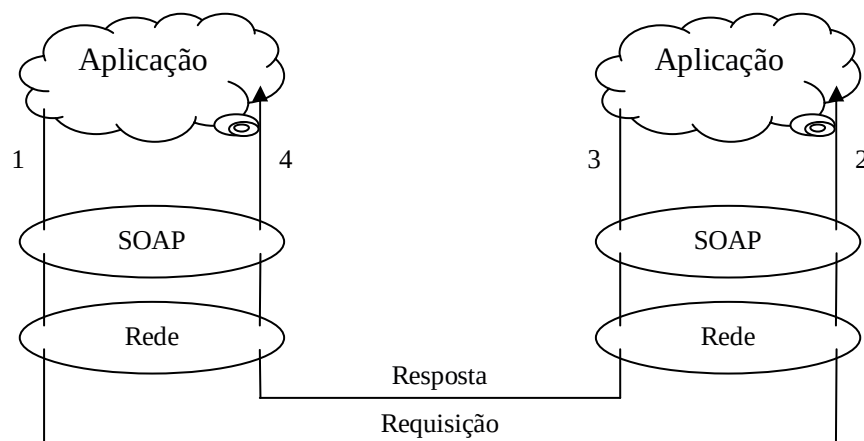
Figura 2.9 – Invocação de um serviço através do protocolo SOAP [Scopel 05].
