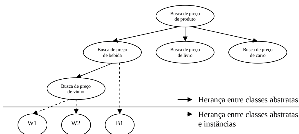
Figura 4.6 – Ontologia do domínio de procura de preço e instancias de serviços. Adaptada de [Zhang 03].
