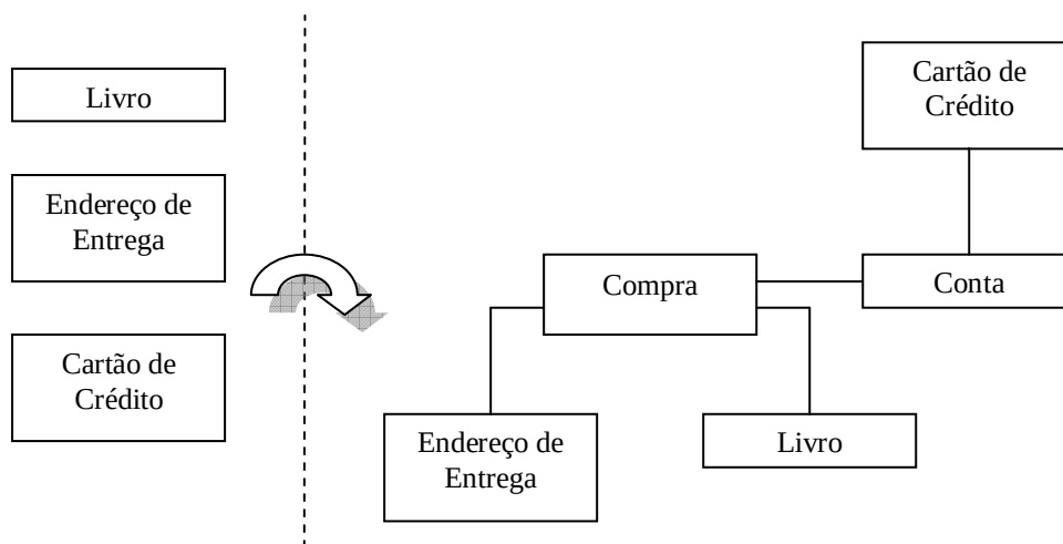
Figura 4.3 – Regra descrevendo a semântica de um web service para venda de livros, a) interface do serviço, b) efeitos da invocação do serviço. Adaptada de [Hausmann 03].
