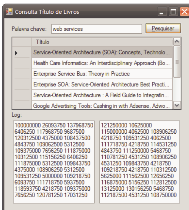
Figura 6.4 – Tela do sistema de consulta de títulos de livros na Amazon.
