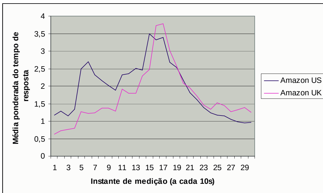
Gráfico 6.3 – Média ponderada do tempo de resposta dos web services da Amazon.
