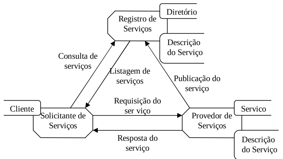
Figura 2.1 – Arquitetura de web services . Adaptada de [Ferris 03].
