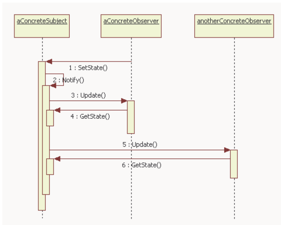
Figura 3.4 – Diagrama de seqüência mostrando a colaboração do padrão observer .
