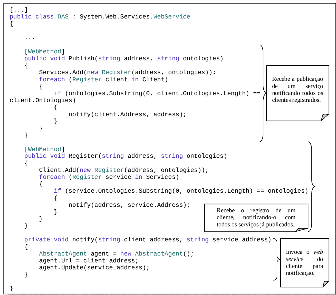
Figura 5.5 – Esqueleto de código do diretório ativo de serviços.
