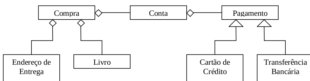
Figura 4.2 – Ontologia para venda de livros. Adaptada de [Hausmann 03].
