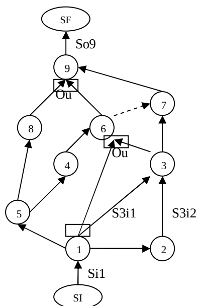
Figura 4.8 – Técnica de composição IMA
