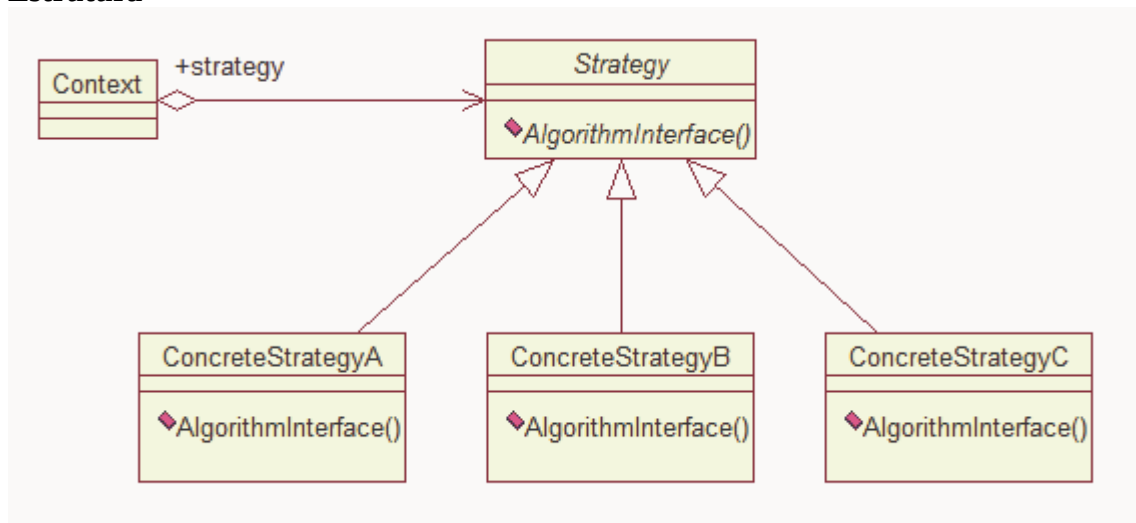
Figura 3.5 – Diagrama de classe UML do padrão strategy [Shalloway 00].
