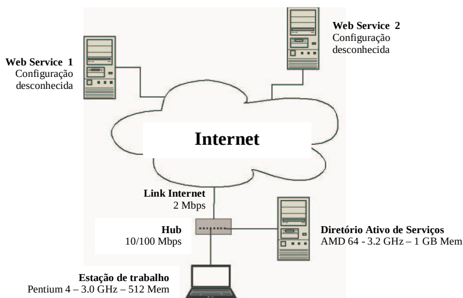
Figura 6.1 – Ambiente de execução
