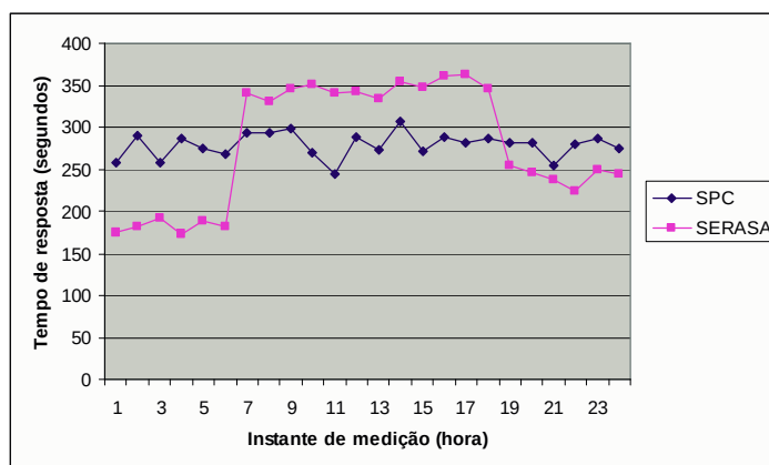
Gráfico 6.1 – Tempo de resposta do SPC e SERASA.
