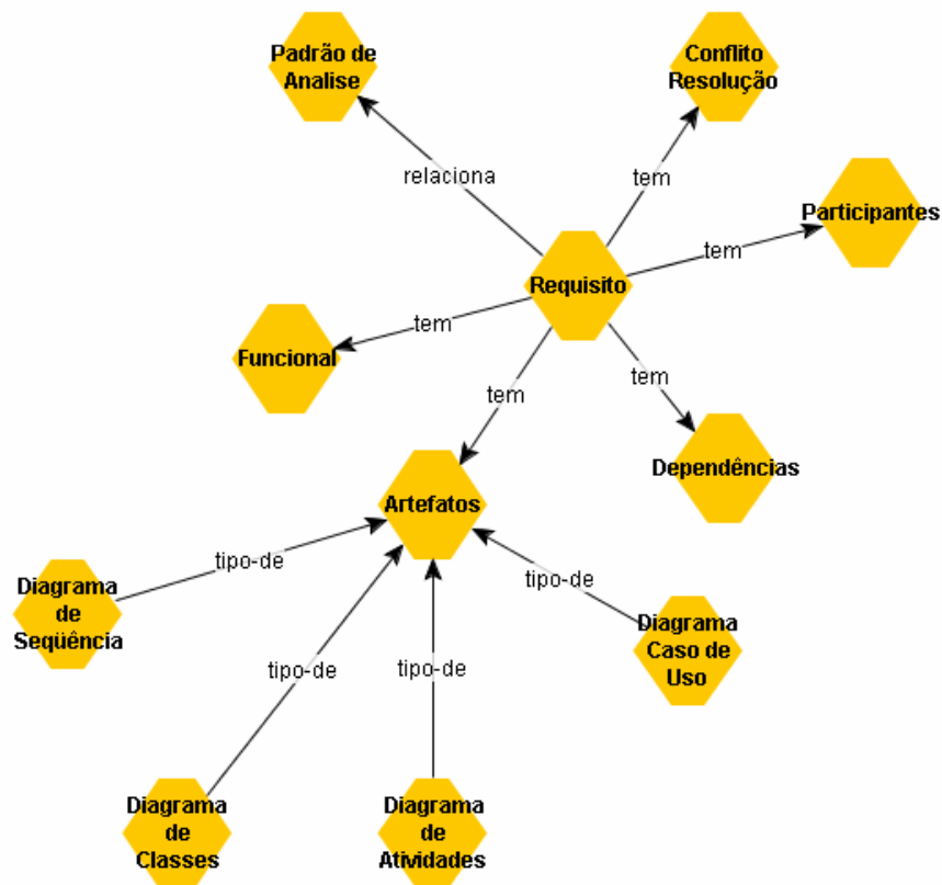
Figura 52: Rede semântica envolvendo requisitos e artefatos
