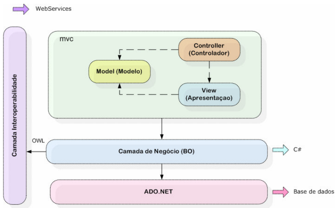
Figura 29: Arquitetura da Ferramenta RPAO
