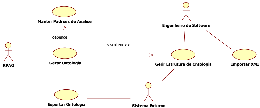
Figura 39: Diagrama de caso de uso Gerar Ontologias
