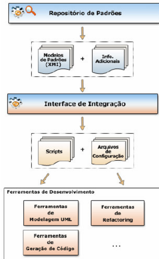
Figura 24: Cenário de Aplicação da Interface de Integração.
