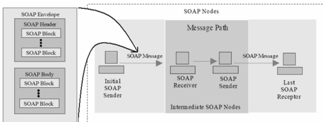
Figura 14: Mensagem SOAP e a navegação entre nodos, adaptado de [HANS 02].
