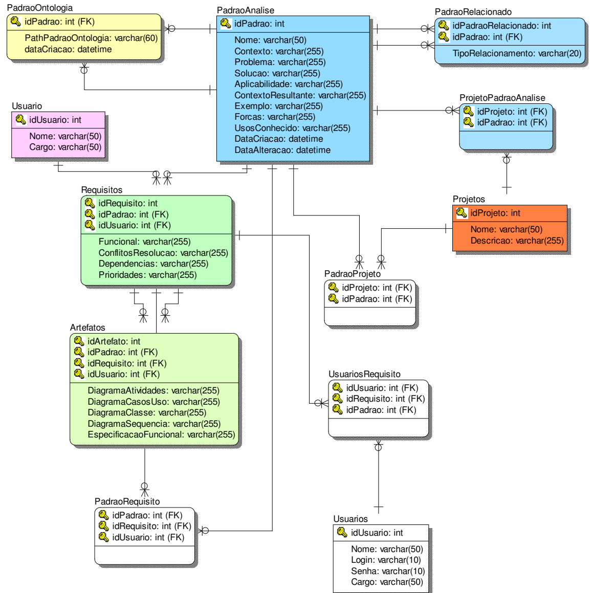
Figura 45: Modelo Relacional (ER).
