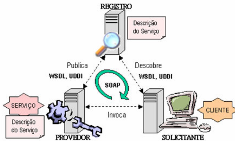
Figura 12: Papéis e tecnologias relacionadas.
