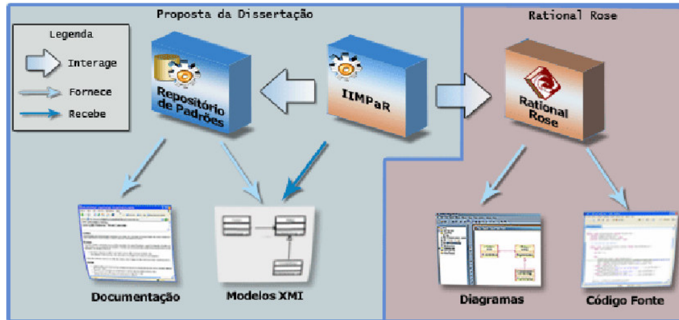
Figura 21: Proposta de Integração do Repositório de Padrões.
