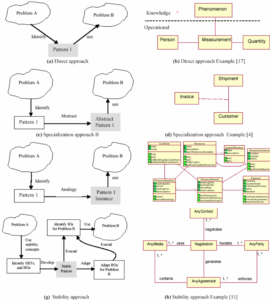
Figura 25: Abordagens de Padrões de Análise.
