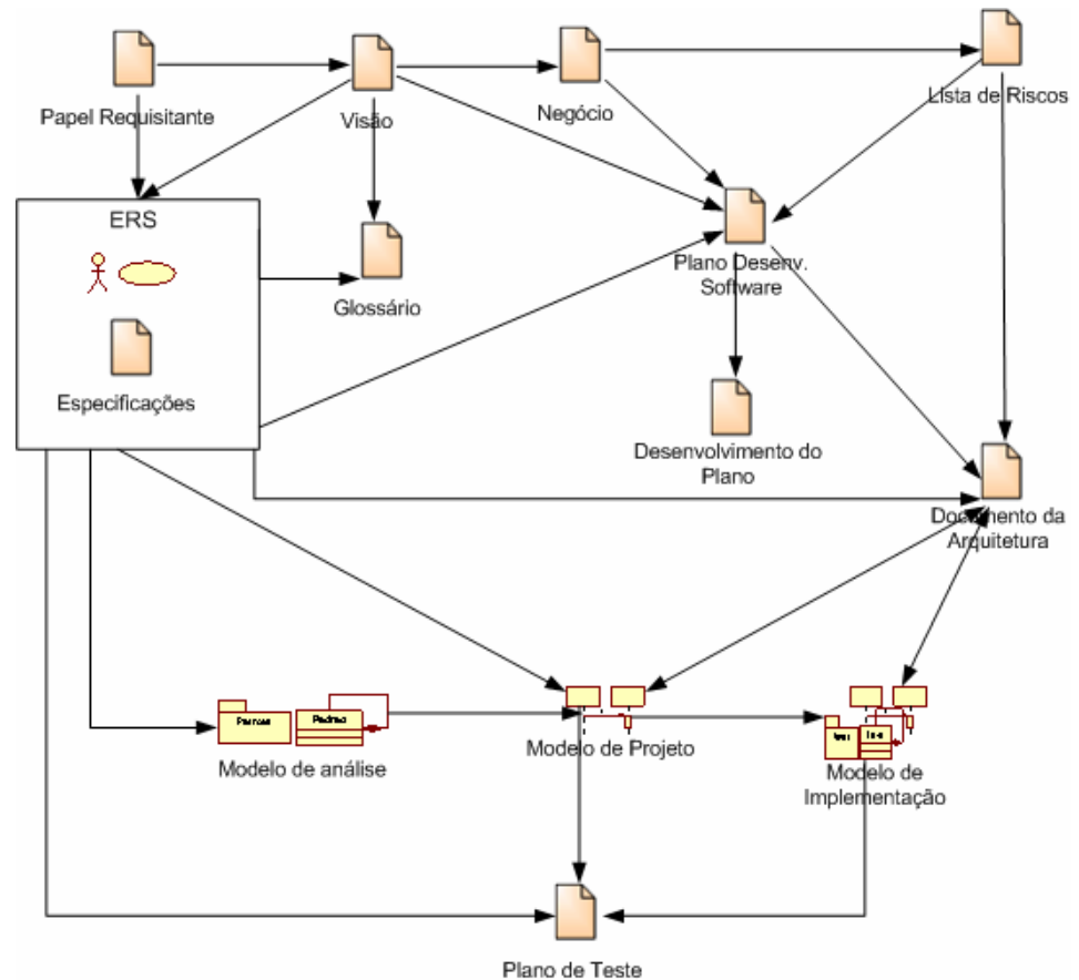
Figura 9: Fluxo de artefatos no RUP.
