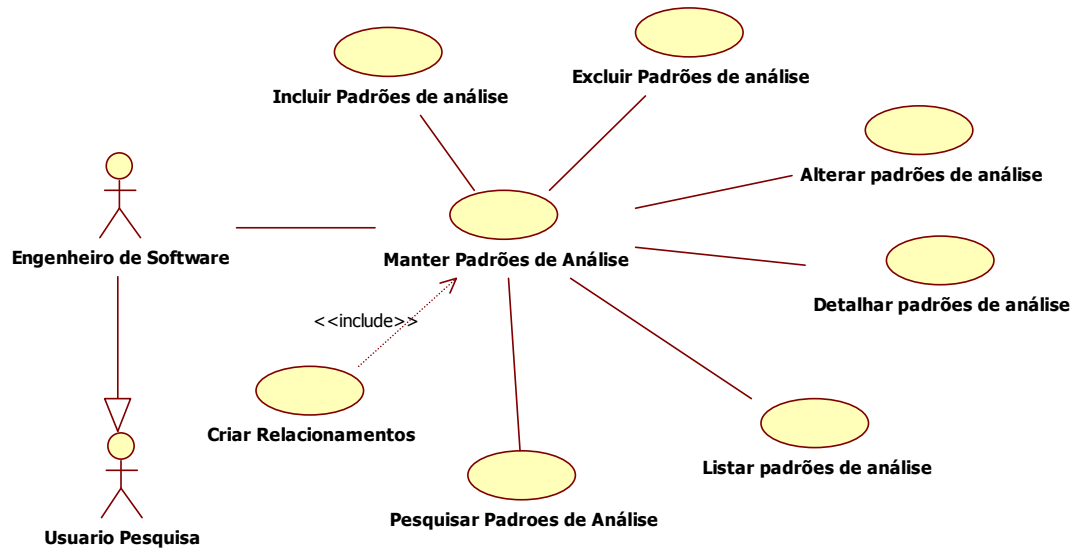
Figura 32: Diagrama de caso de uso manter padrões de análise.
