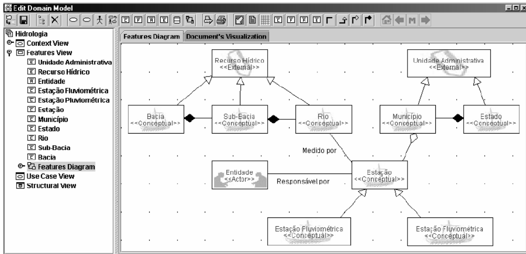
Figura 19: Modelo de features do domínio Hidrologia.
