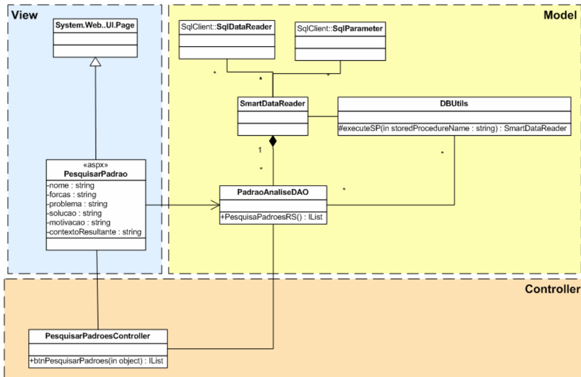
Figura 28: Padrão MVC para o RPAO.
