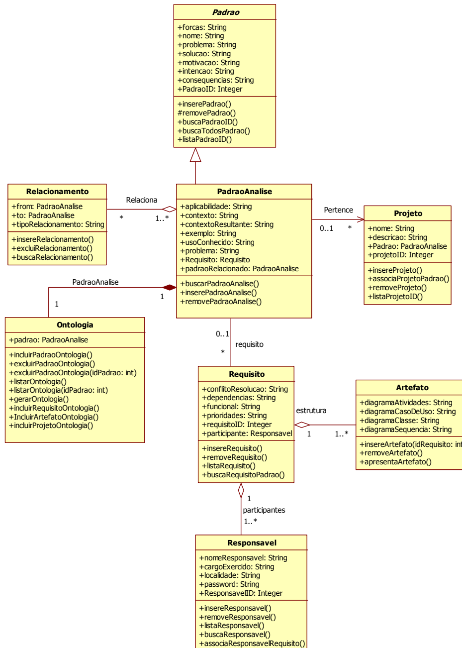
Figura 43: Diagrama de Classes de Análise RPAO.
