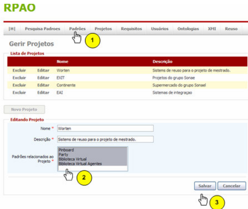
Figura 60: Criação de um padrão de análise
