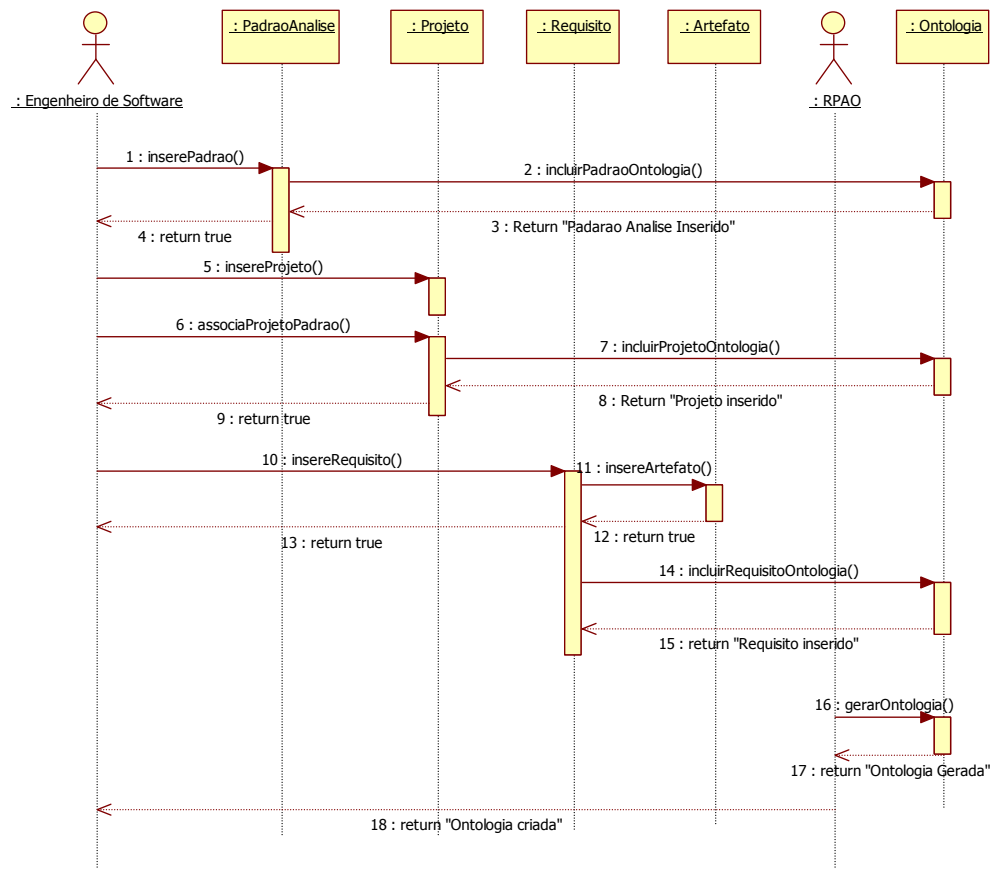
Figura 44: Diagrama de sequência inclusão de Padrão de Análise.
