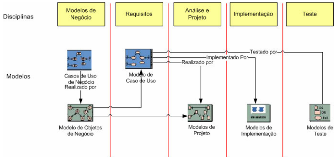
Figura 8: Workflows e Modelos.
