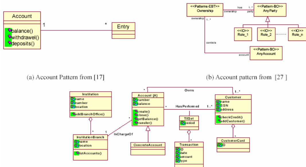
Figura 26: Diferente estrutura do padrão Conta.
