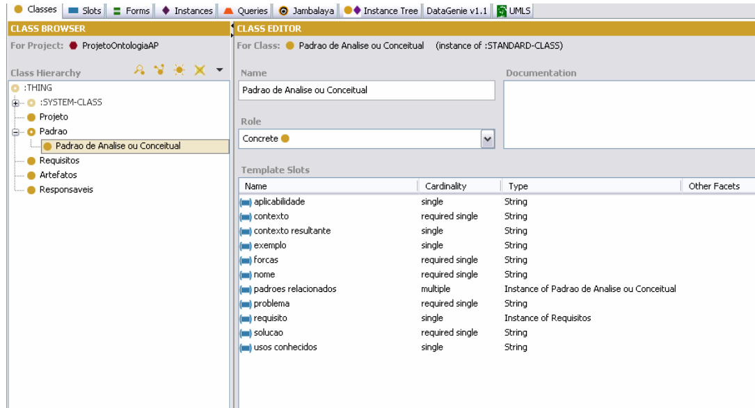
Figura 53: Hierarquia de Classes da Onto-APattern.
