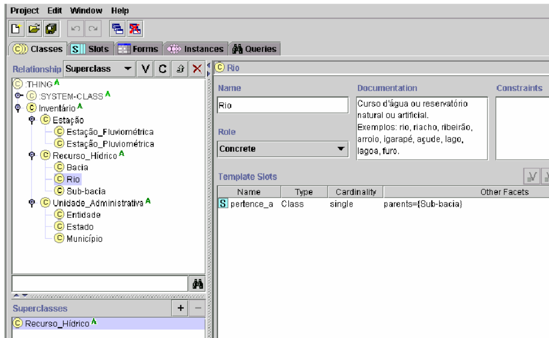
Figura 18: Ontologia do projeto Hidrologia.
