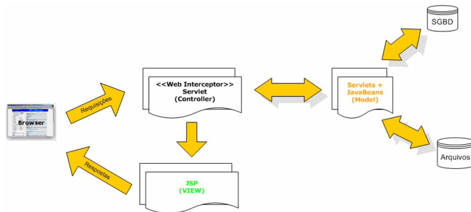
Figura 23: Arquitetura do Repositório de Padrões.
