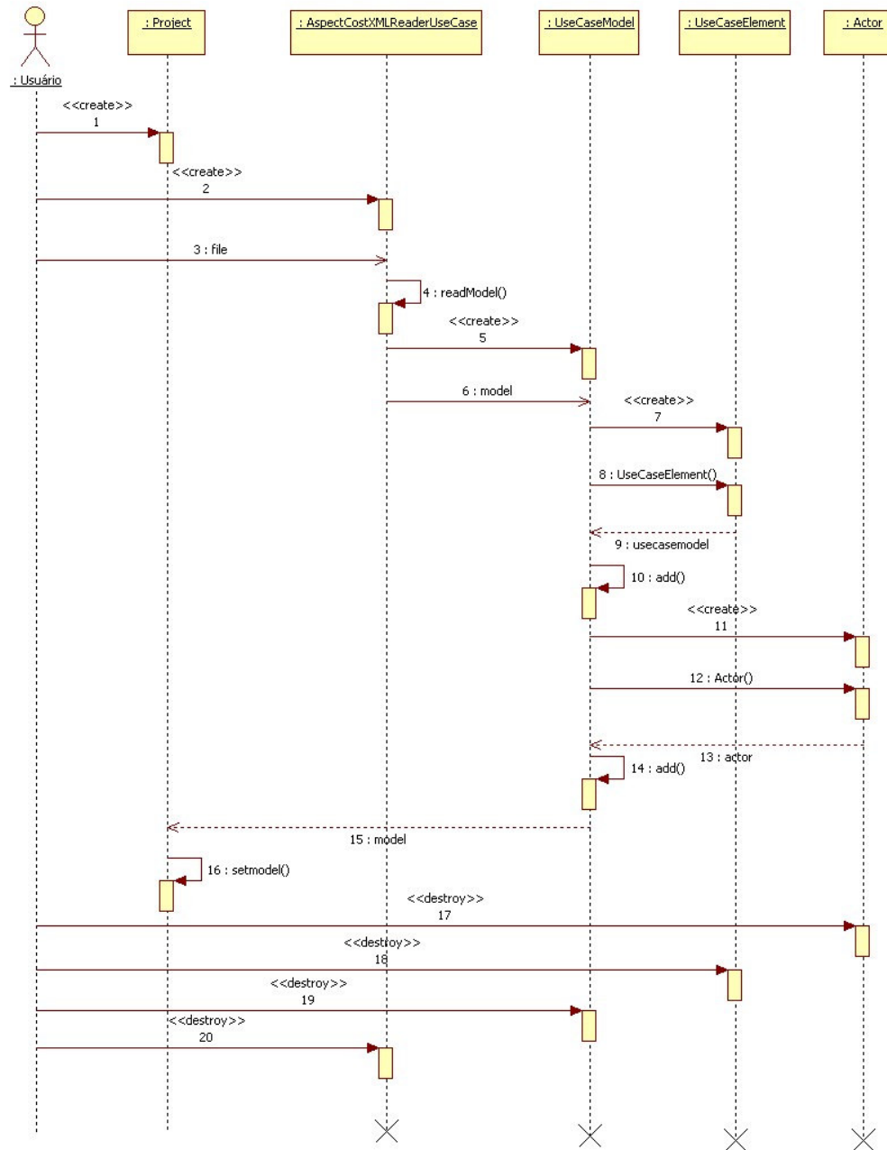
Figura 15 : Diagrama de sequência – Ler Arquivo
